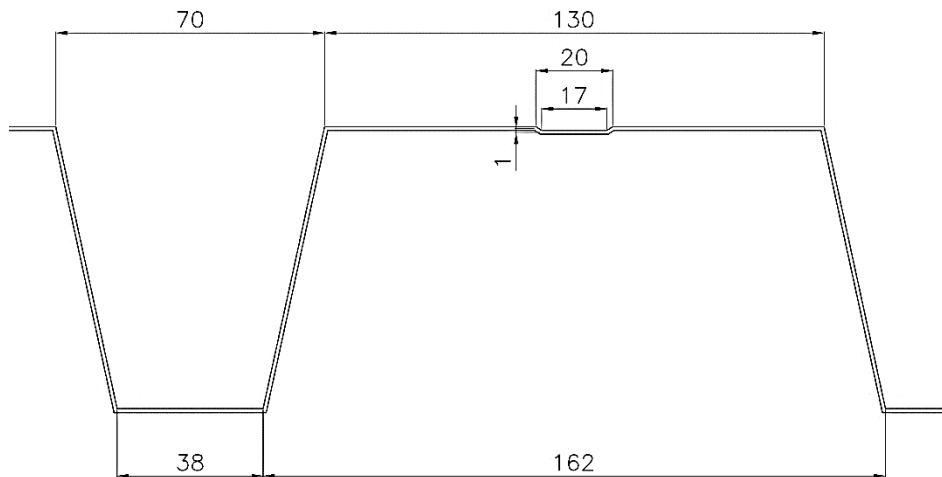
Figura 6: Lamiera R/C 400, distanze fra i rulli con superficie di riferimento superiore.
