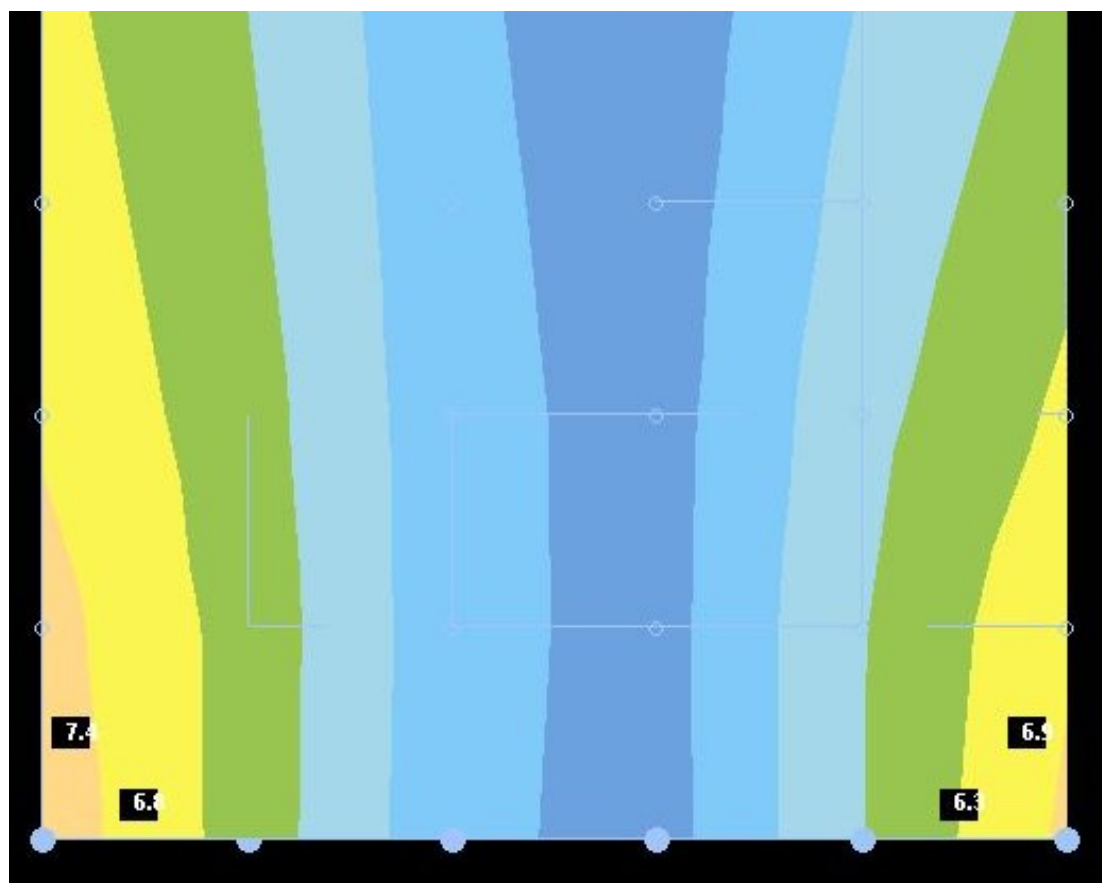
Figura 93: Sisma Ancona, combinazione SLUSISY, \sigma_{max} nel setto 20.
