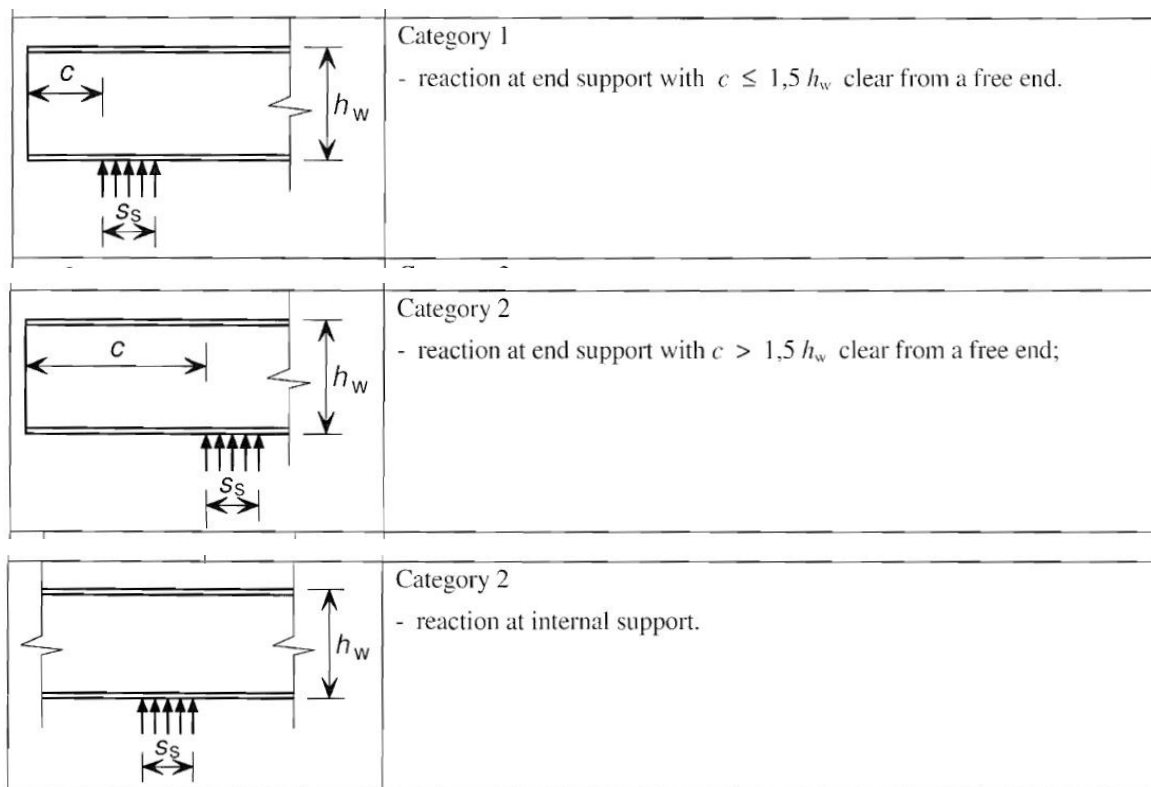
Figura 18: Schemi e dimensioni per la classificazione degli appoggi laterali e intermedi secondo il capitolo 6.1.7.3 dell'EN 1993-1-3.
