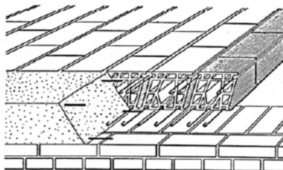
Figura 12: Solaio tipo "SAP".
